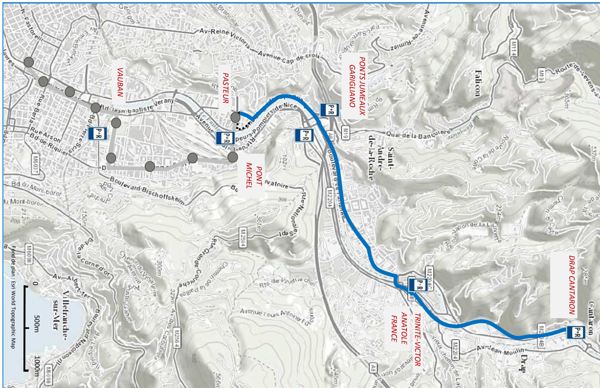
Tracé du tram-train du sud vers le nord : Arrêt T1 Pasteur/rue Maurice Maccario/ av. Joseph Raybaud/Bd de l’Ariane/Av Emile Rippert/Bd de l’Ariane/Pont Anatole France/voie ferrée Nice-Breil/Gare de Drap-Cantaron.
